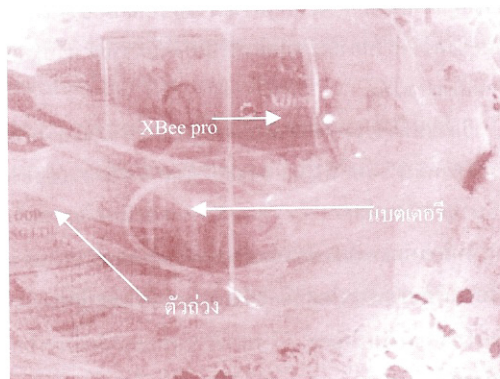
รูปที่ 5 โหนดย่อยที่ใช้ต่อกับตัวตรวจจับ
