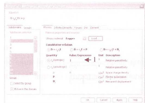
รูปที่ 9 กำหนดคุณสมบัติของทองแดง
