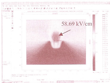
รูปที่ 12 การกระจายสนามไฟฟ้ามุม 90 องศา
