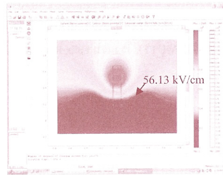
รูปที่ 15 การกระจายสนามไฟฟ้ามุม 30 องศา
