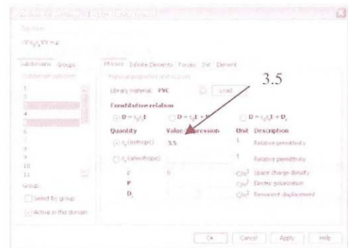
รูปที่ 8 กำหนดคุณสมบัติของท่อ PVC
